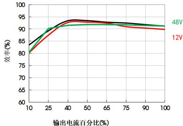
效率Vs输出负载 (Vin=230VAC)
