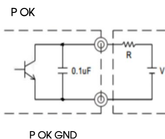
图 1 电源正常的内部回路（集电极开路的方法） (最大吸入电流 10mA, 最大电压 30V)
