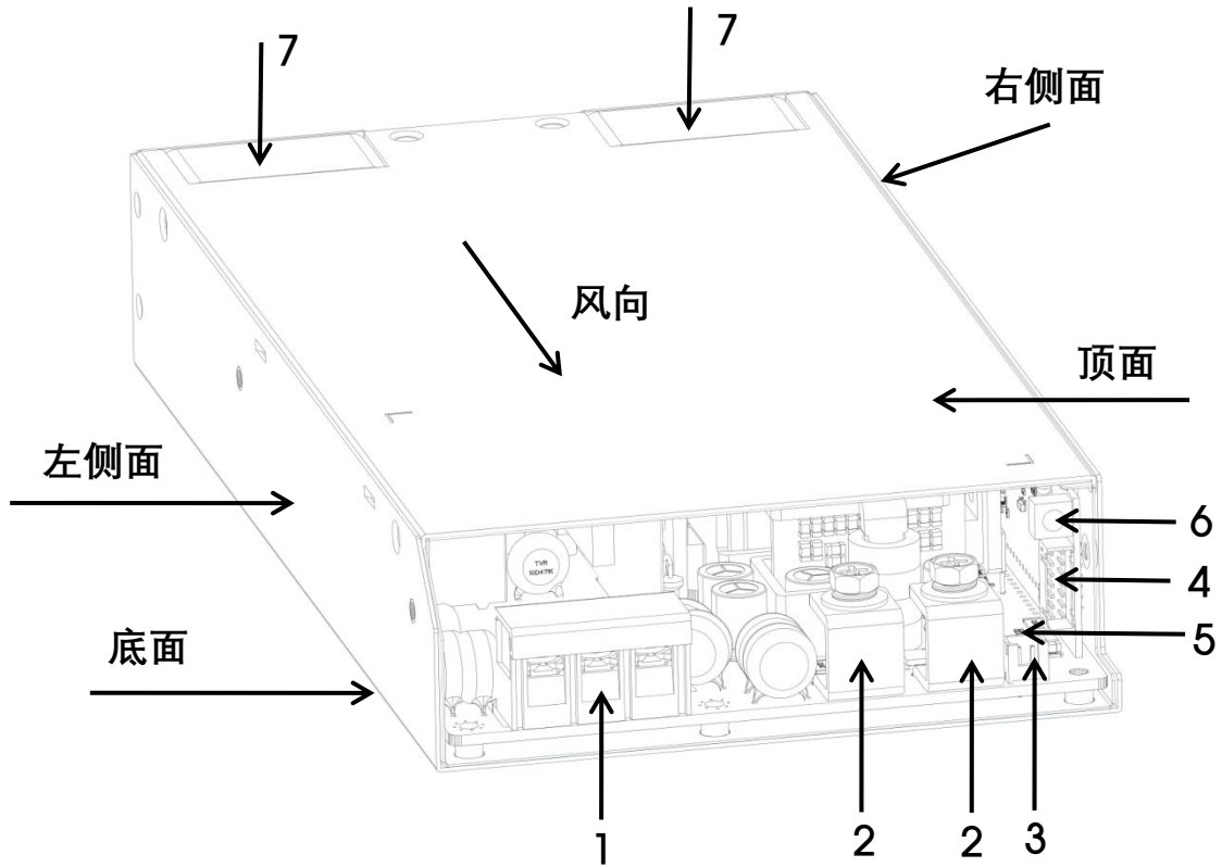
图 1: AMF1500-Bxx(-QQ)外观信息
