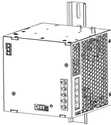
旋转安装位置(90° Z-轴)
