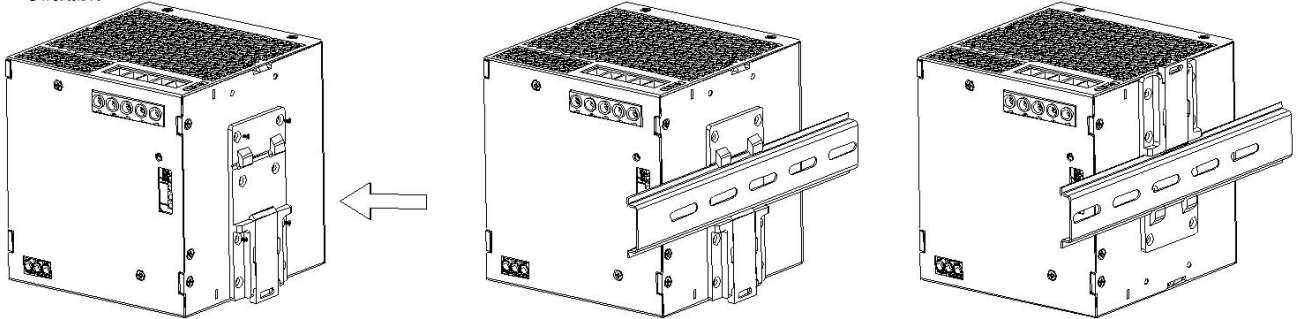
② 安装通用DIN导轨适配器 (侧面反装, 需撕标签纸)
