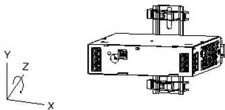
旋转安装位置(180° Z-轴)
