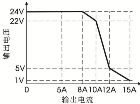
过流保护示意图(Typ.)
