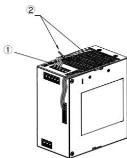
①端子接上连接线后，铺设和对齐 连接线； ②通过外壳两侧的缺口，用电缆捆 扎条，固定连接线。
