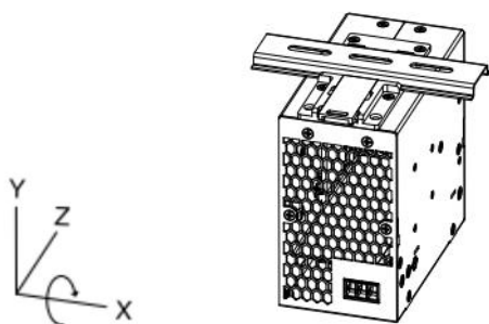
旋转安装位置(270° X-轴)
