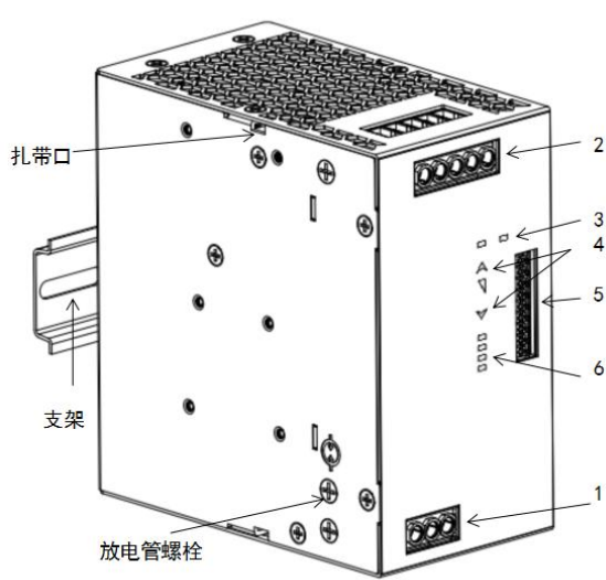
图 1：AIHF480-Bxx 外观信息
