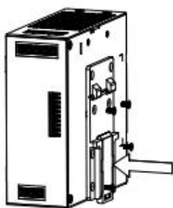
① 安装通用DIN导轨适配器 (侧面正装，需撕标签纸)
