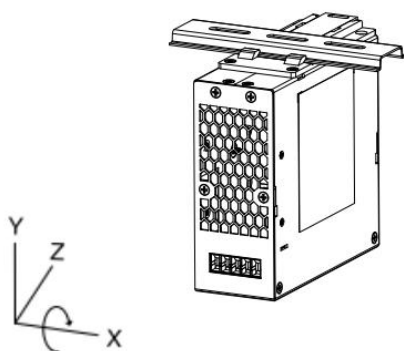
旋转安装位置(270° X-轴)
