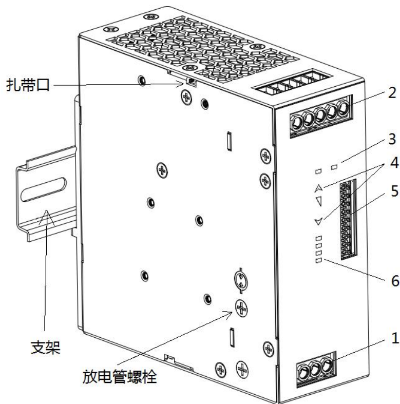
图 1: AIHF240-Bxx 外观信息
