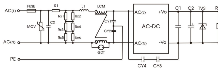
图 3：I 类设备推荐电路
