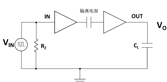
图 2 上升/下降时间&传输延时测试电路、波形
