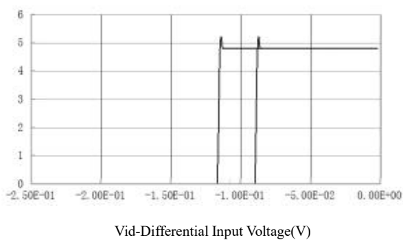
图12 接收器输出电压 VS 差分输入电压
