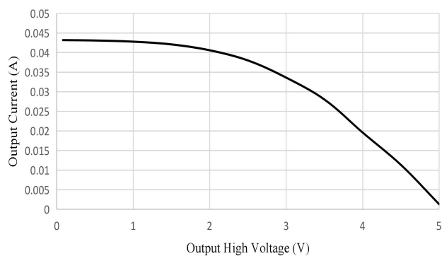
图2 输出电流 VS 接收器输出高电压
