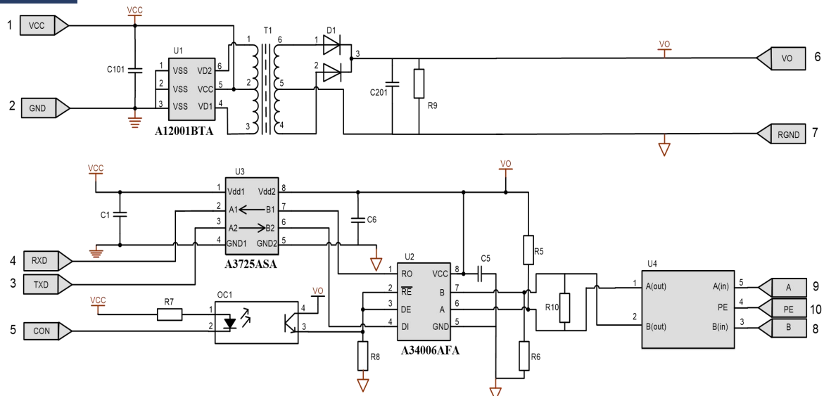
图 26 用于 UART 转 RS485 信号的隔离应用电路原理图
