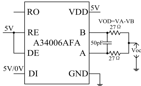
图 16 驱动器测试电路，VOD、VOC 无共模负载
