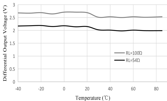
图7 驱动器差分输出电压 VS 温度
