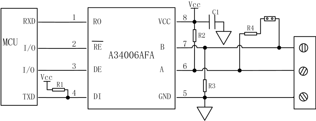
典型应用电路 2（典型设计）
