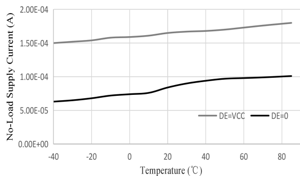
图1 供电电流 (空载) VS. 温度
