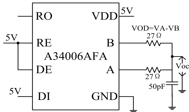
图 18 驱动器 VOC 输出测试电路及波形
