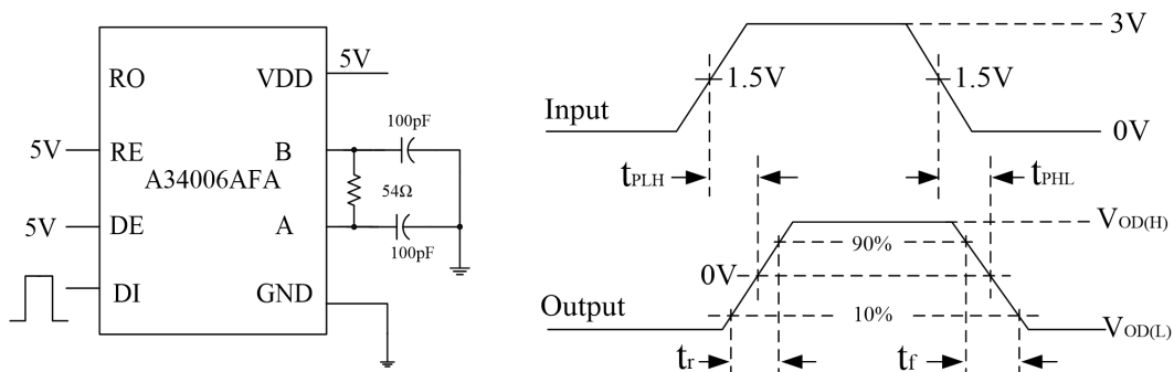
图 19 驱动器开关测试电路及波形
