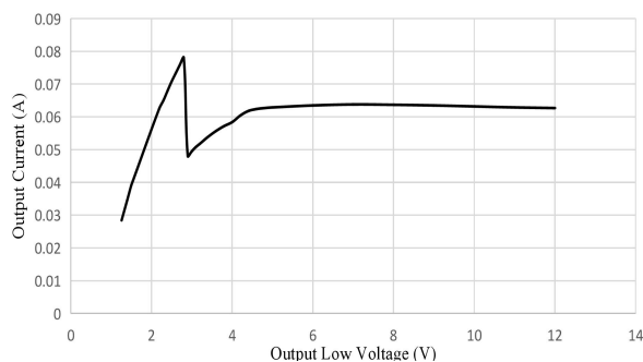
图9 输出电流 VS 发射器输出低电压
