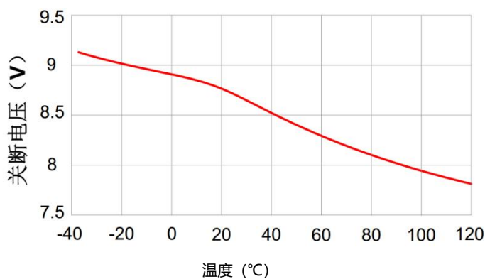
图三：关断电压和温度关系
