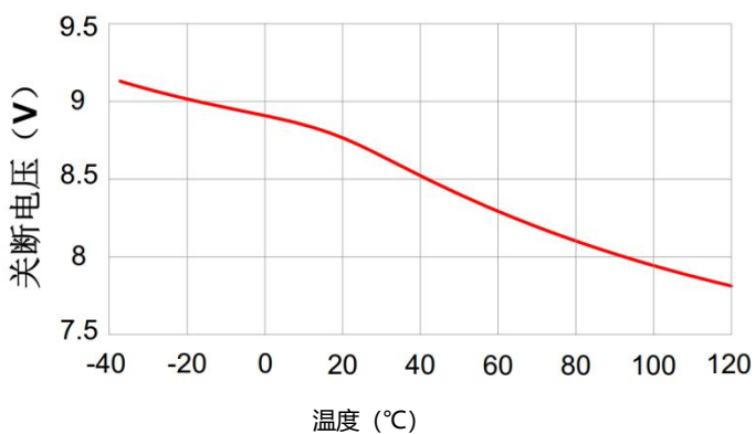
图四：线损电流和温度关系
