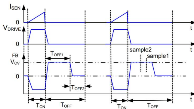
图 7: 恒流原理
