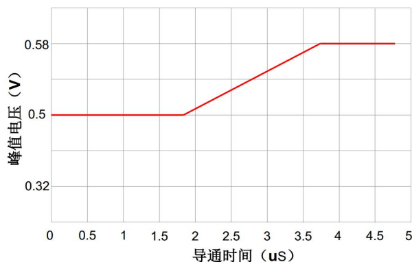
图 8: 峰值电流补偿
