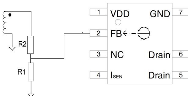
图 9: 输出线损补偿原理图
