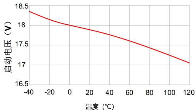
图二：启动电压和温度的关系
