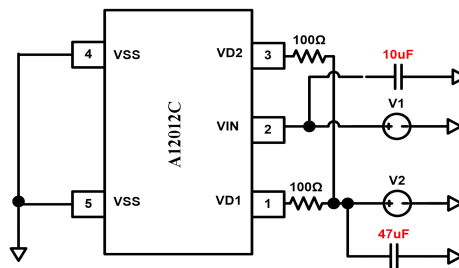
图 7 开关特性测试电路原理图
