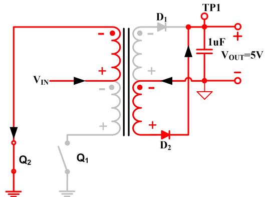
图 9 推挽变换器的开关周期 2
