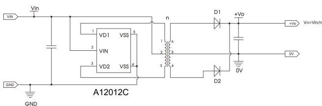
图 15 拓展电路 1
