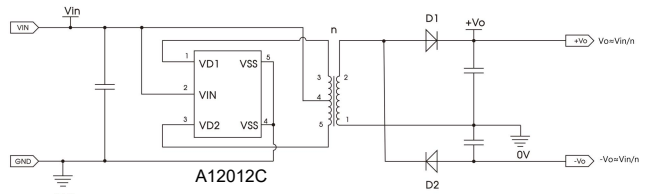
图 16 拓展电路 2
