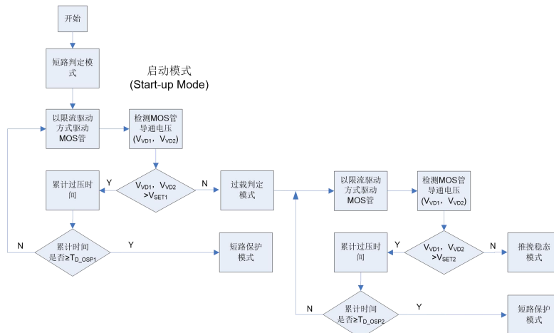
图 12 启动模式流程图
