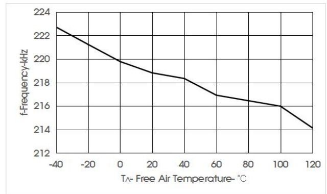
图 4 MOS 管开关频率 VS 环境温度
