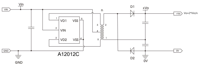
图 17 拓展电路 3
