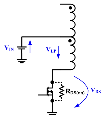
图 11 自适应的正温度系数的 R_{ds(on)}
