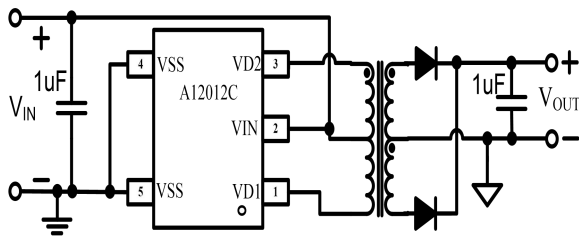
图 5 功能曲线测试电路原理图
