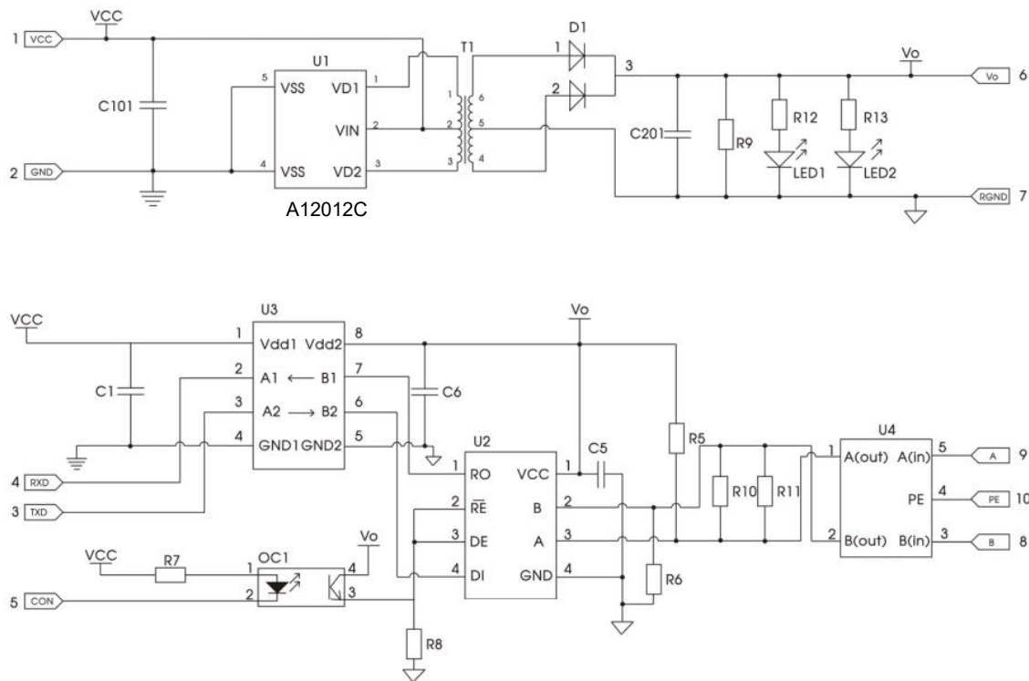
图 19 应用电路一
