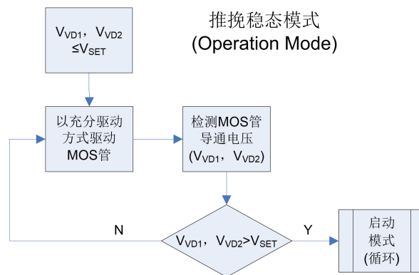
图 13 推挽稳态模式流程图
