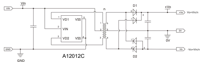
图 16 拓展电路 2
