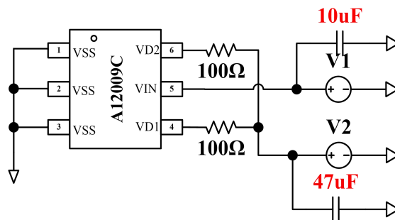
图 7 开关特性测试电路原理图
