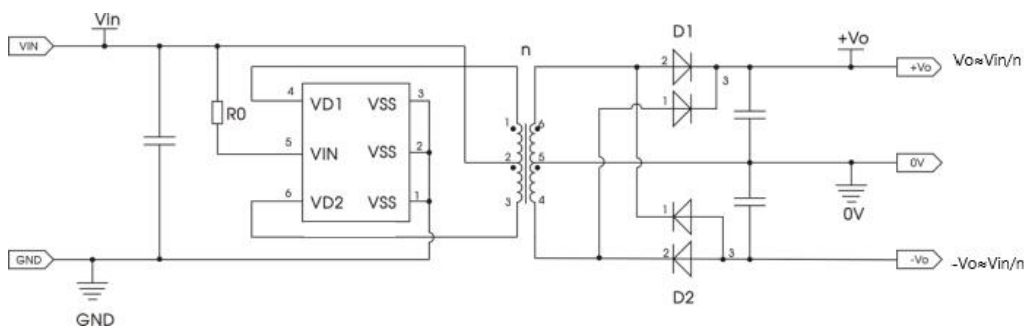
图 16 拓展电路二
