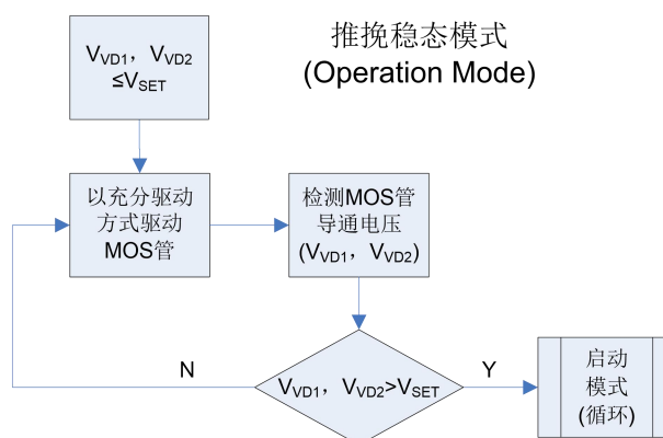
图 13 推挽稳态模式流程图
