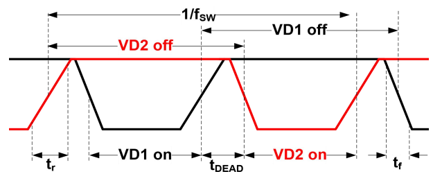
图 6 电路时序图
