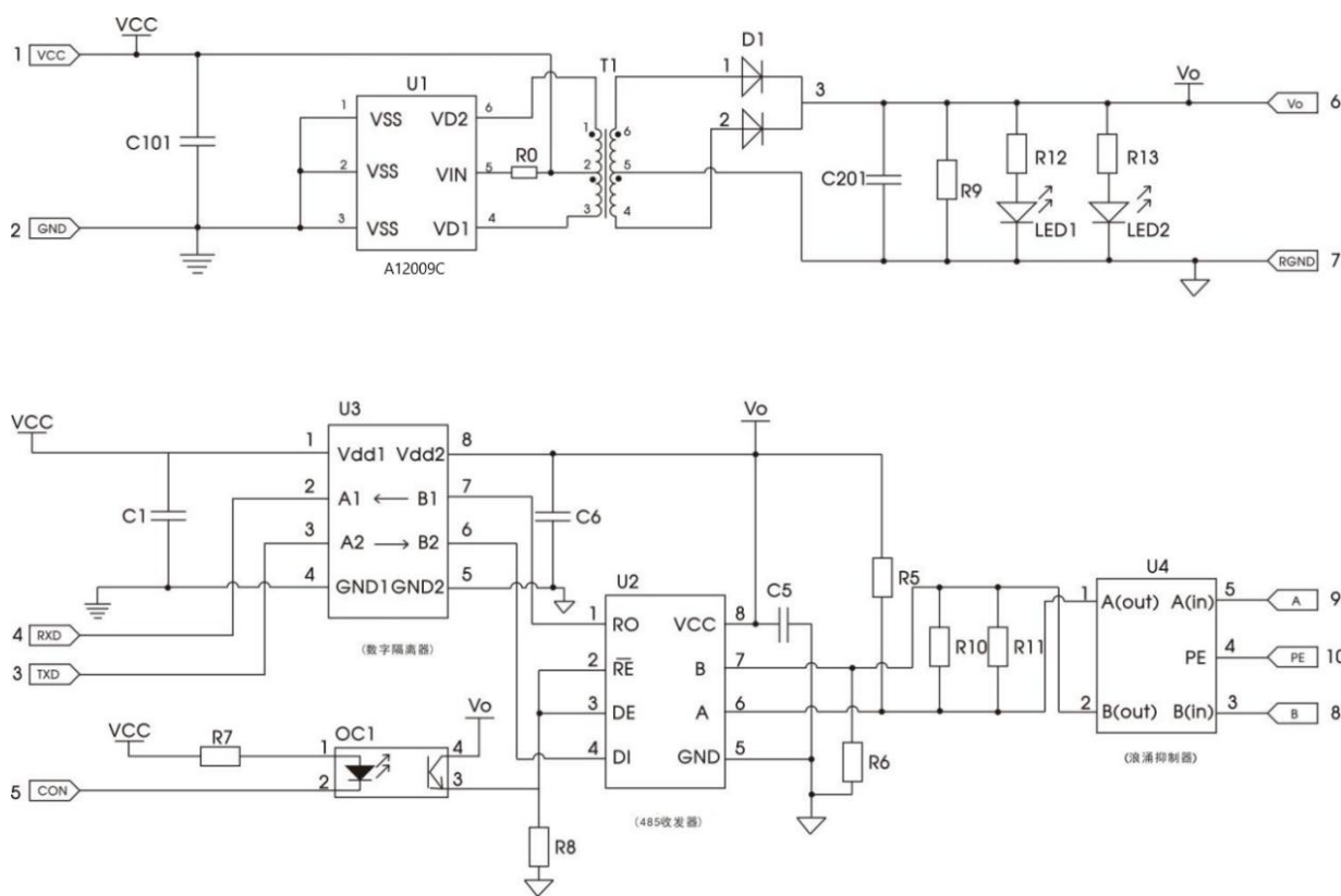
图 19 应用电路一
