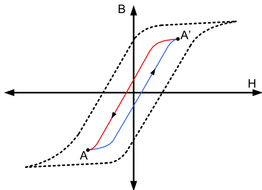
图 10 磁化曲线
