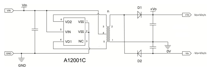
图 18 拓展电路四
