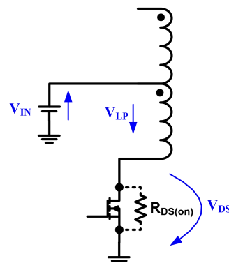
图 11 自适应的正温度系数的 R_{DS(on)}
