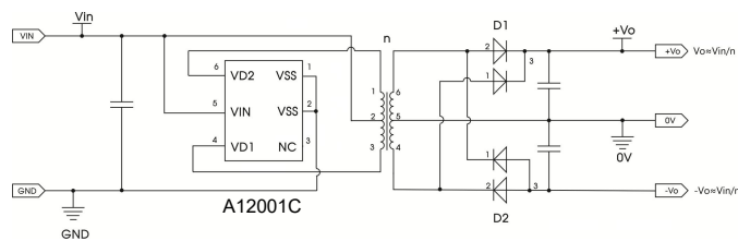
图 16 拓展电路二
