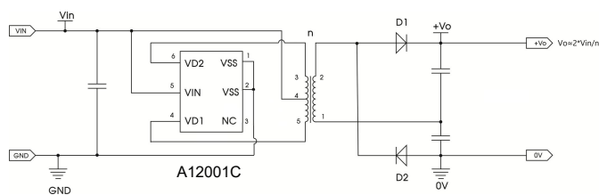
图 17 拓展电路三
