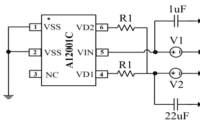
图 7 开关特性测试电路原理图
