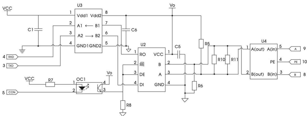
图 19 应用电路一
