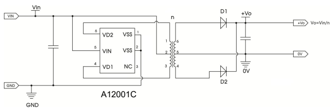
图 15 拓展电路一
