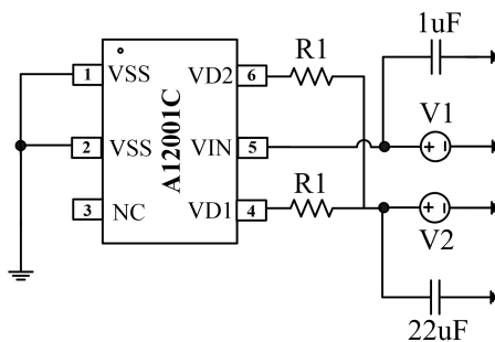
图 7 开关特性测试电路原理图
