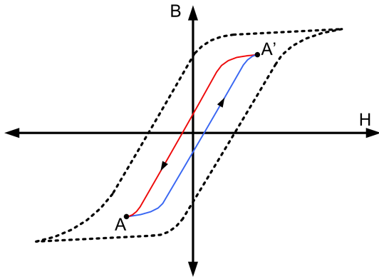
图 10 磁化曲线
