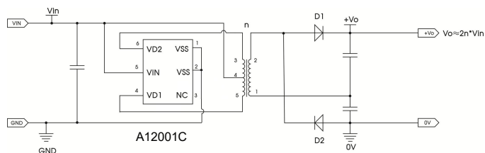
图 17 拓展电路三
