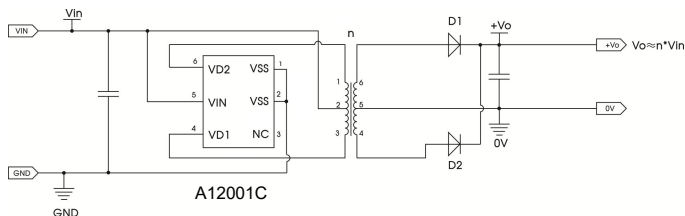
图 15 拓展电路一
