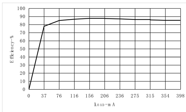
图 3 效率 VS 负载电流
