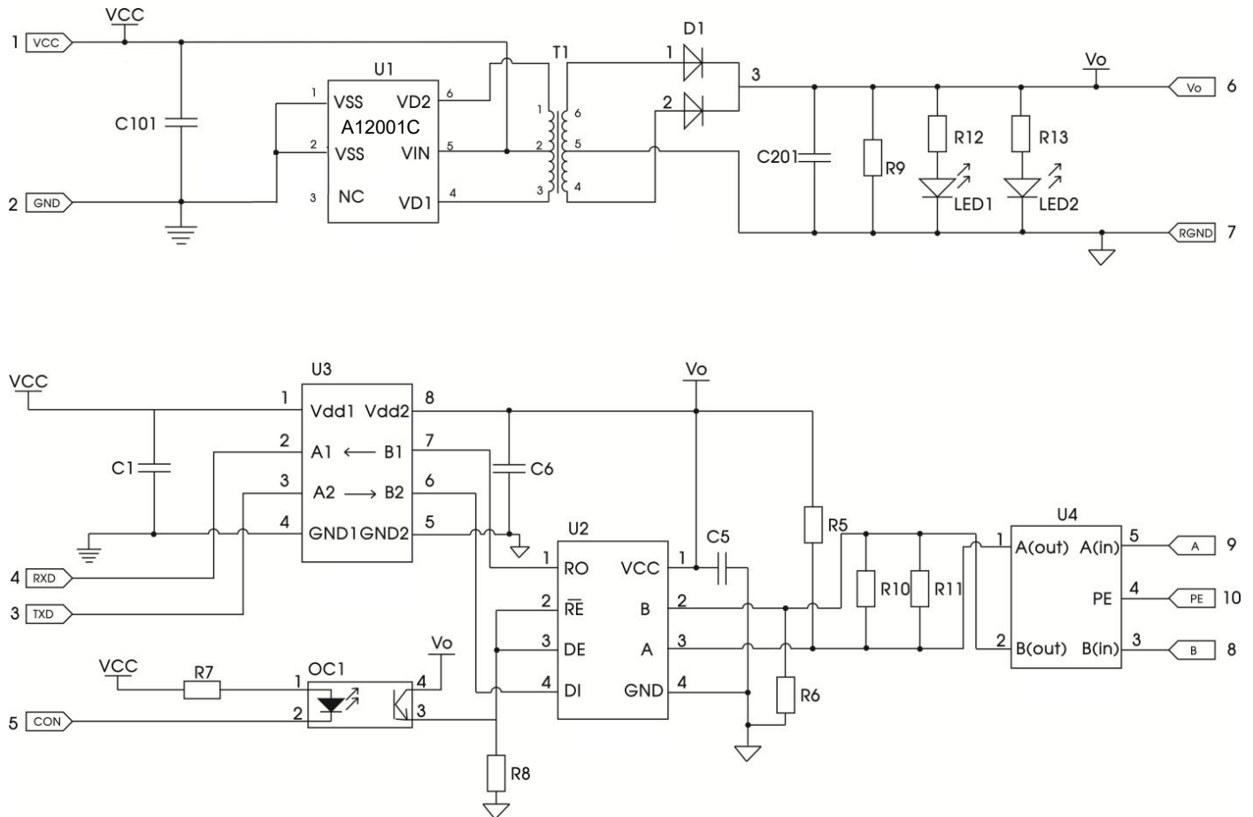
图 19 应用电路一
