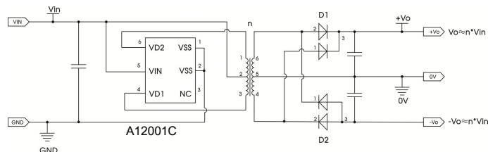
图 16 拓展电路二
