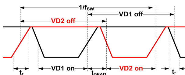
图 6 电路时序图
