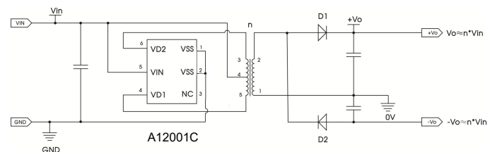
图 18 拓展电路四
