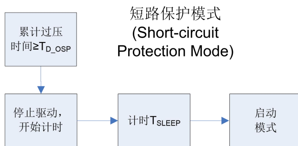
图 14 短路保护模式流程图
