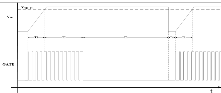
图 20 输出短路时 V_{FR} 与 GATE 的时序图
