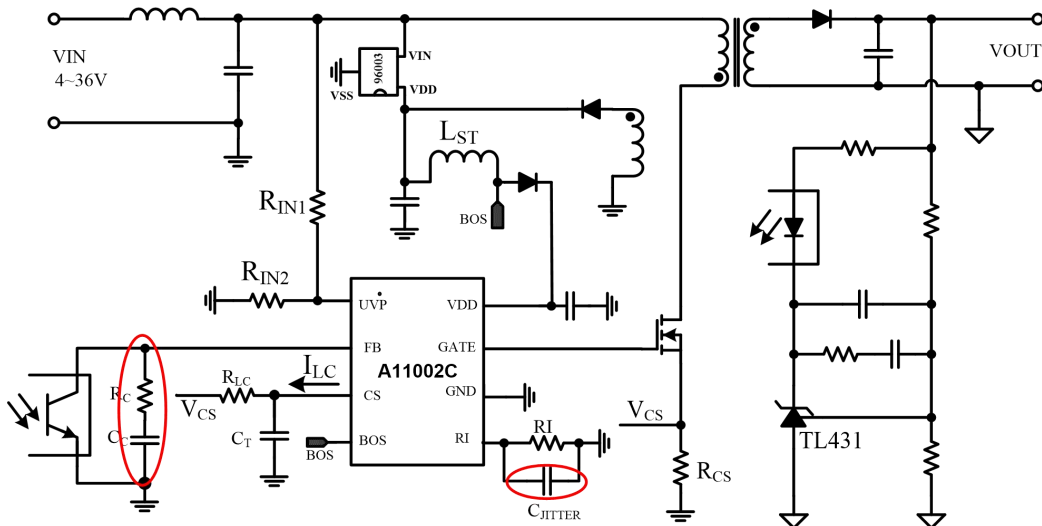
图 23 典型应用电路 3，外接 DCDC 启动芯片 96003（SOT-23 封装）实现低压到高压全范围输入，红色圈部分器件可选
