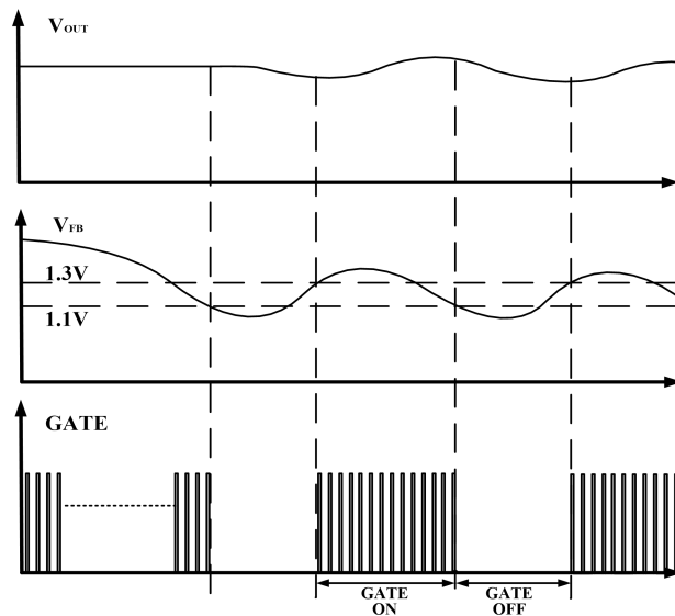
图 17 间歇 BURST 模式工作相关波形
