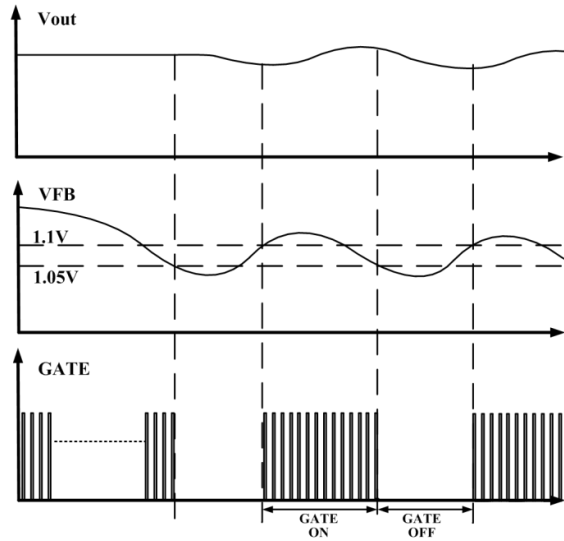
图 16 间歇工作模式时序图
