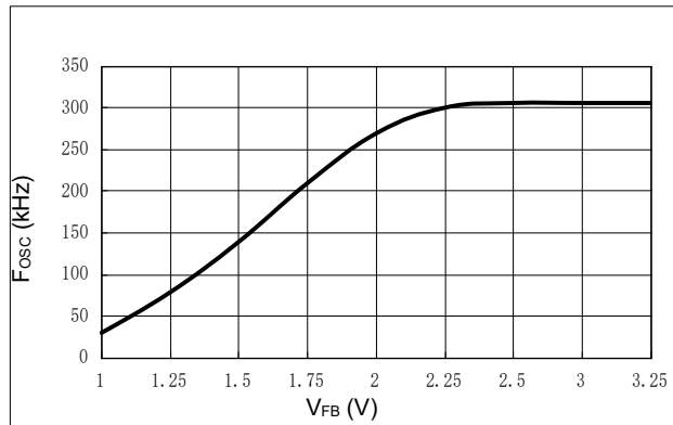
图 6 工作频率 VS V FB 电压
