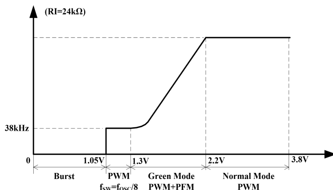
图 15 FB 引脚电压与输出频率的关系
