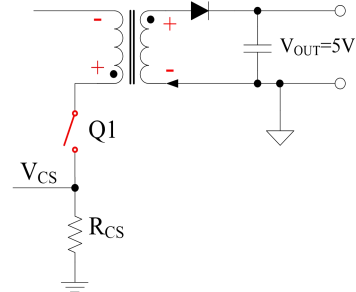
图 14 反激变换器的开关断开
