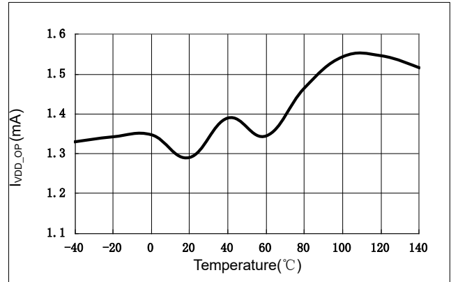
图4 芯片工作电流 VS 温度
