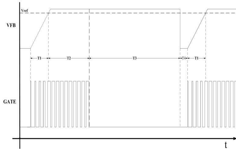
图 17 输出短路时 VFB 与 GATE 的时序图
