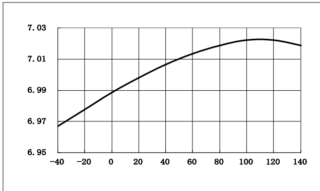
图 1 欠压锁定撤销 VS 温度
