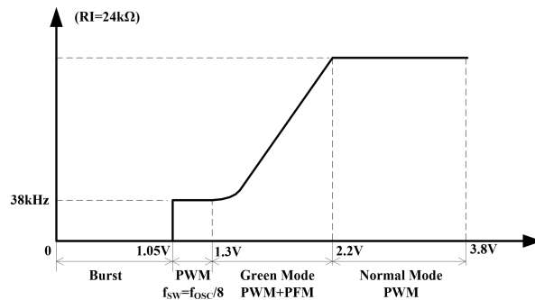
图 15 FB 引脚电压与输出频率的关系
