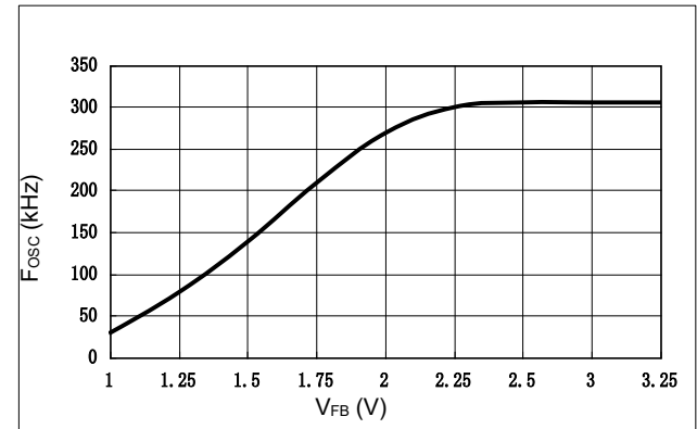
图6 工作频率 VS VFB 电压
