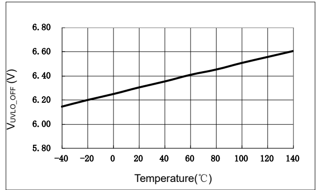
图 2 欠压锁定开启 VS 温度
