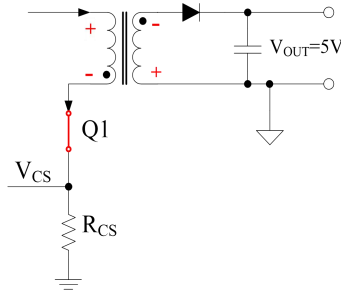
图 13 反激变换器的开关闭合
