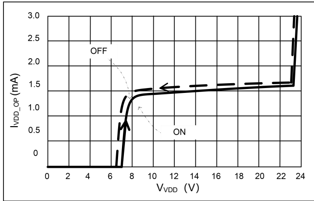
图3 芯片工作电流 VS VDD 电压
