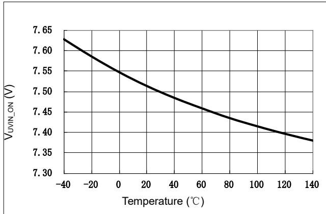
图 9 输入欠压撤销电压 VS 温度
