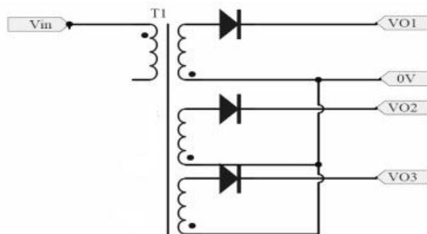
图 18 拓展电路, 多路输出
