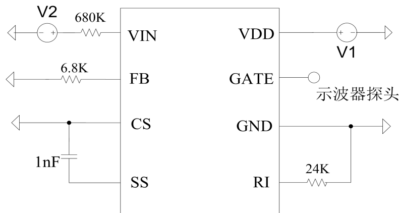
图 12 电学特性测试电路原理图
