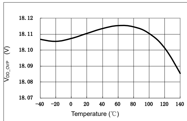
图11 VDD过压保护电压 VS 温度
