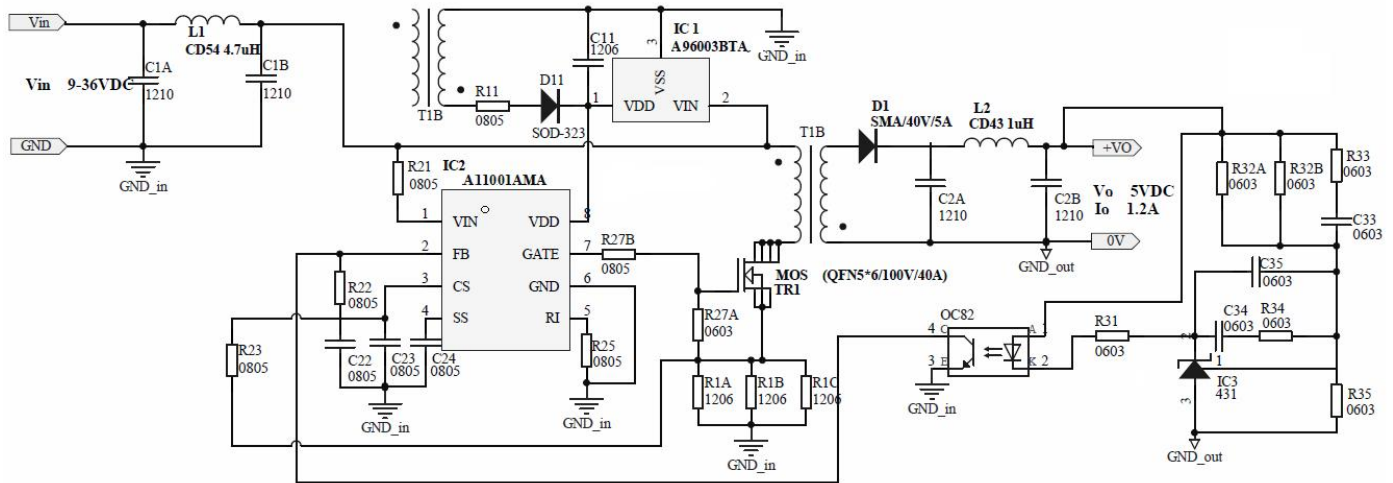
图 19 应用电路
