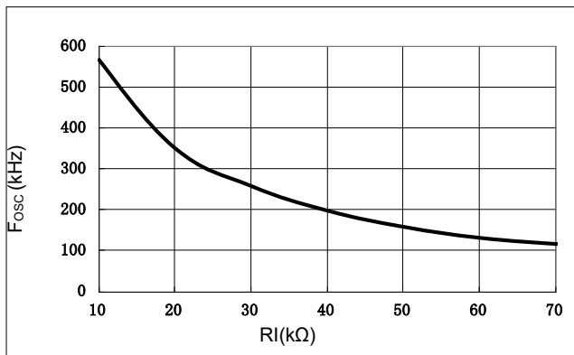
图7 工作频率 VS RI 脚电阻
