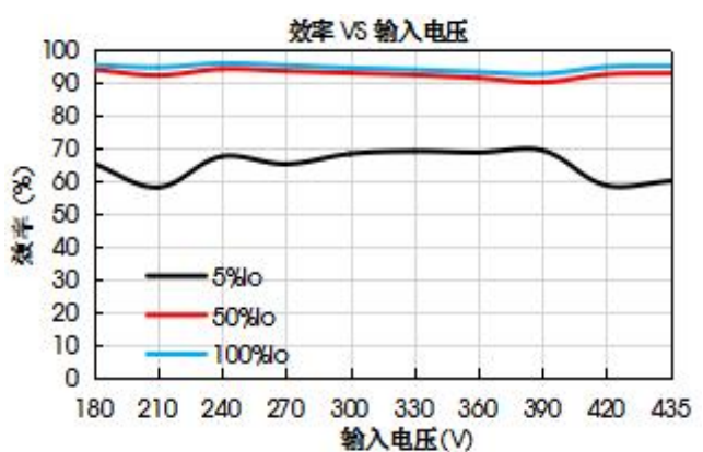
VFB600-F3D48 效率VS输入电压
