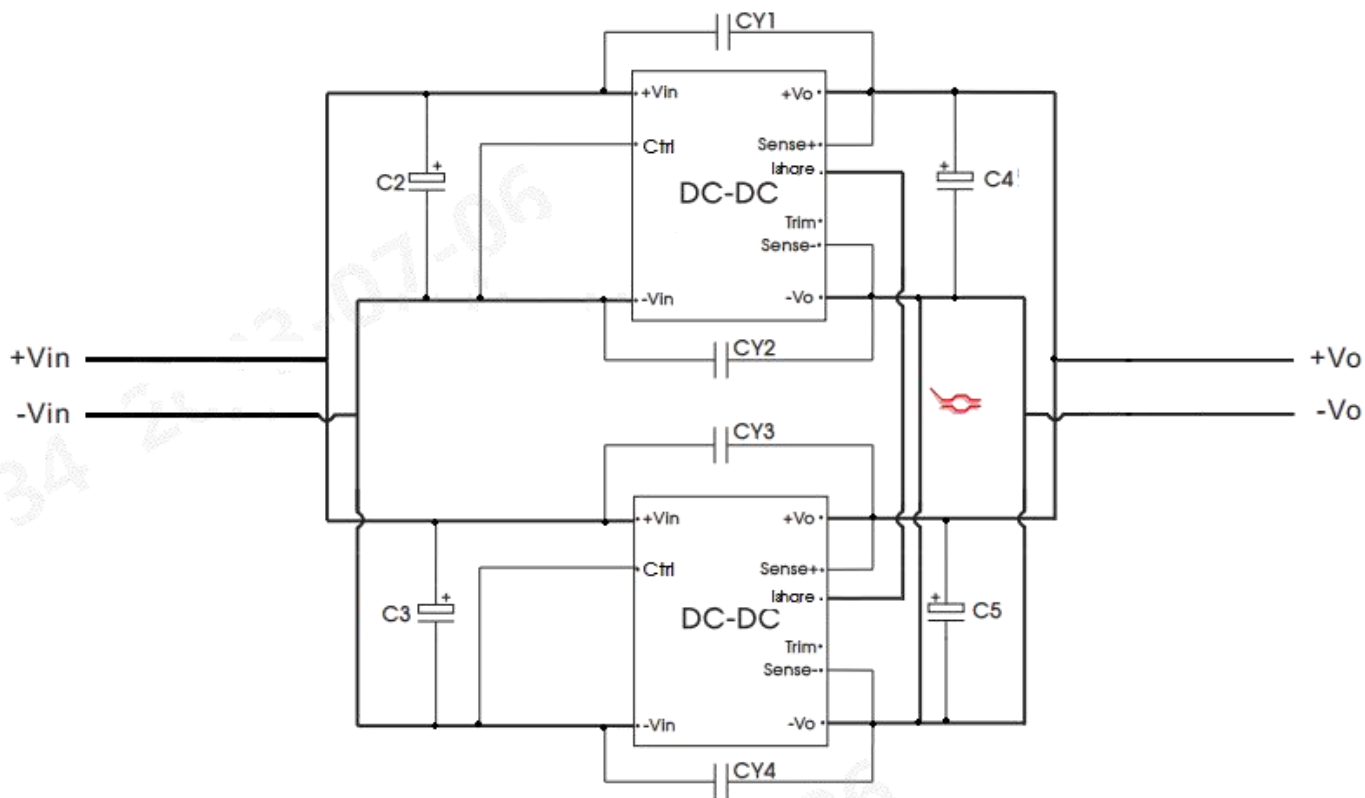
图 10 并联均流接线图
