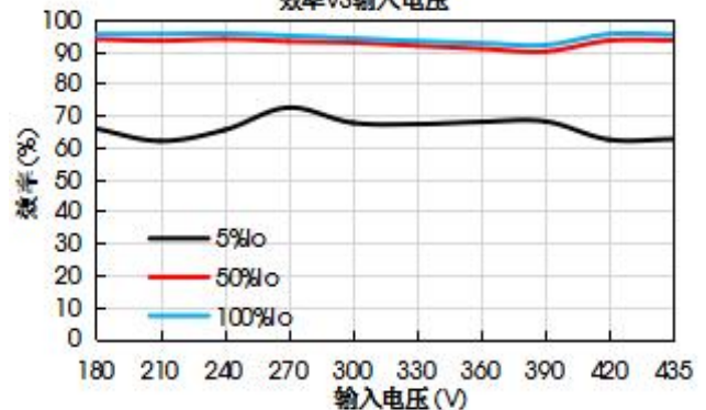
VFB600-F3D48 效率VS输入电压
