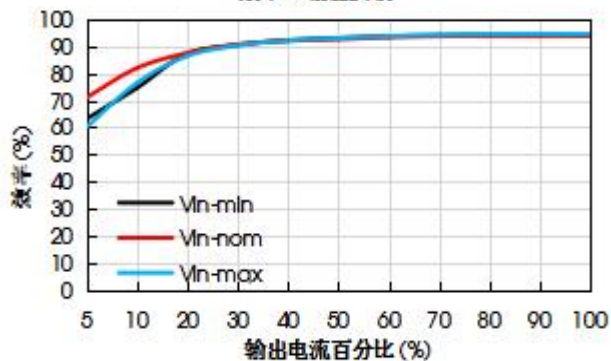
VFB600-F3D24 效率VS输出负载
