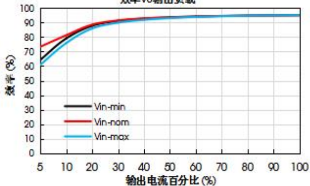
VFB600-F3D28 效率VS输出负载
