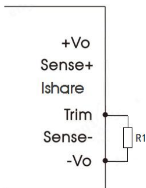
图 7 Trim 的使用电路
