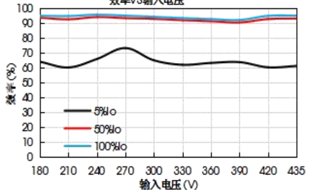
VFB600-F3D28 效率VS输入电压
