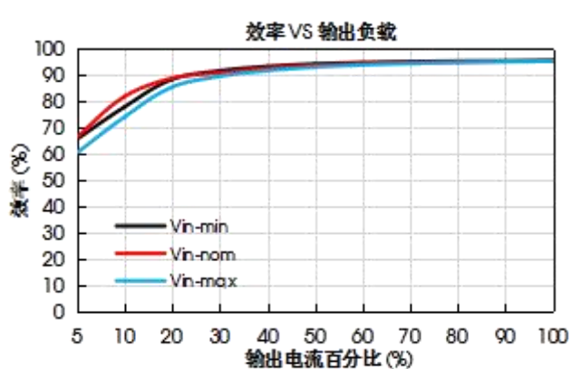
VFB600-F3D48 效率VS输出负载
