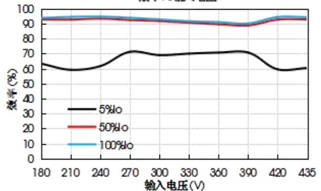
VFB600-F3D24 效率VS输入电压
