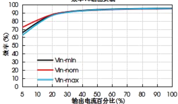
VFB600-F3D48 效率VS输出负载
