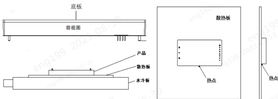
图 11 产品热点图
