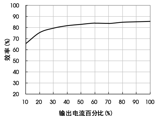
效率Vs输出负载 (标称输入)
